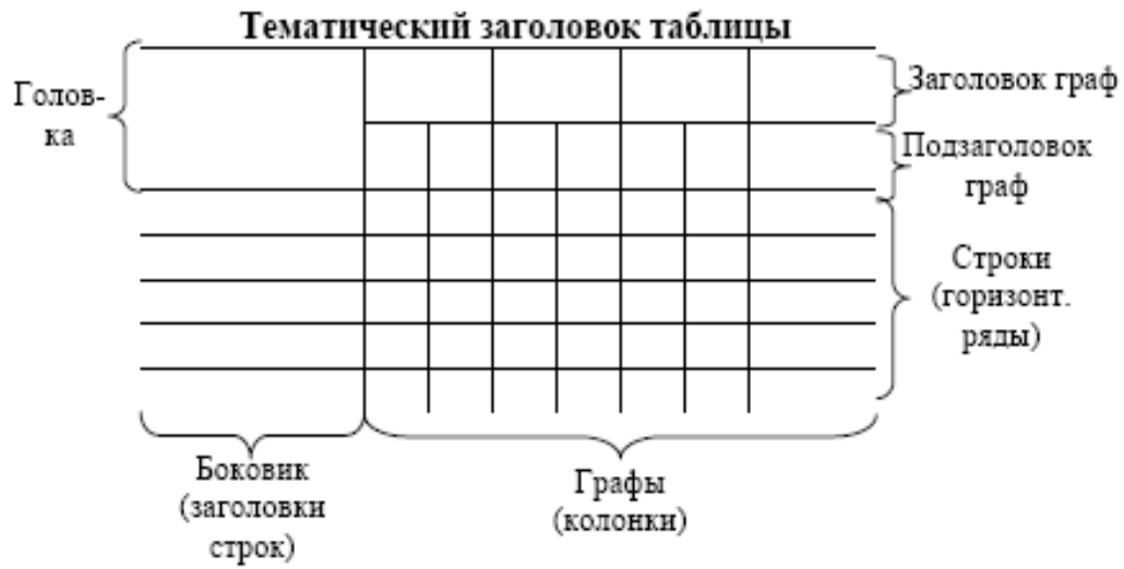
Рисунок 1 – Структура таблицы
